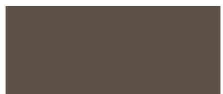
Lignite
